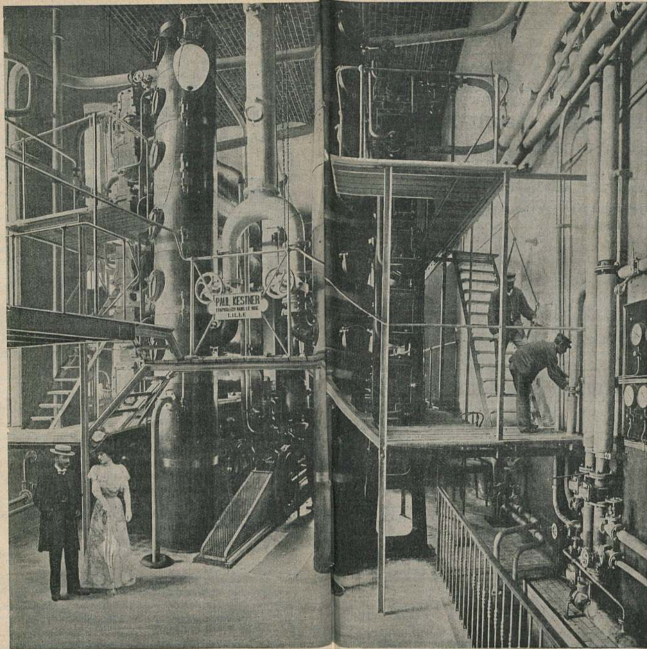
L A Salle d'évaporation. — Appareil concentrateur à double effet, pour l'extraction des sels de Vichy-État. — A la sortie de cet appareil l'eau concentrée au degré voulu est conduite dans une chaudière d'évaporation, où, sous l'influence du vide et d'un brassage continu, tous les sels contenus dans l'eau sont précipités.
