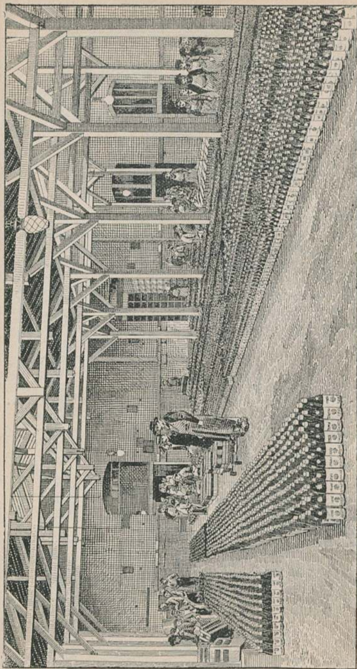
CHANTIER D'EMBALLAGE. — Après l'embouteillage, les bouteilles sont de nouveau amenées à la gare d'emballage, où après avoir reçu les étiquettes, elles sont emballées et mises sur wagons. — La production s'élève souvent à 70,000 bouteilles dans la même journée.
